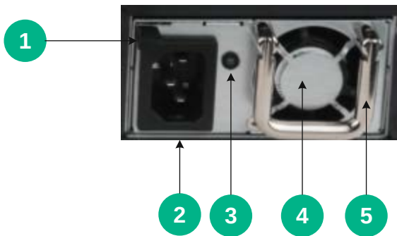
图A-5 R2A-BV0350 交流电源模块正视图
