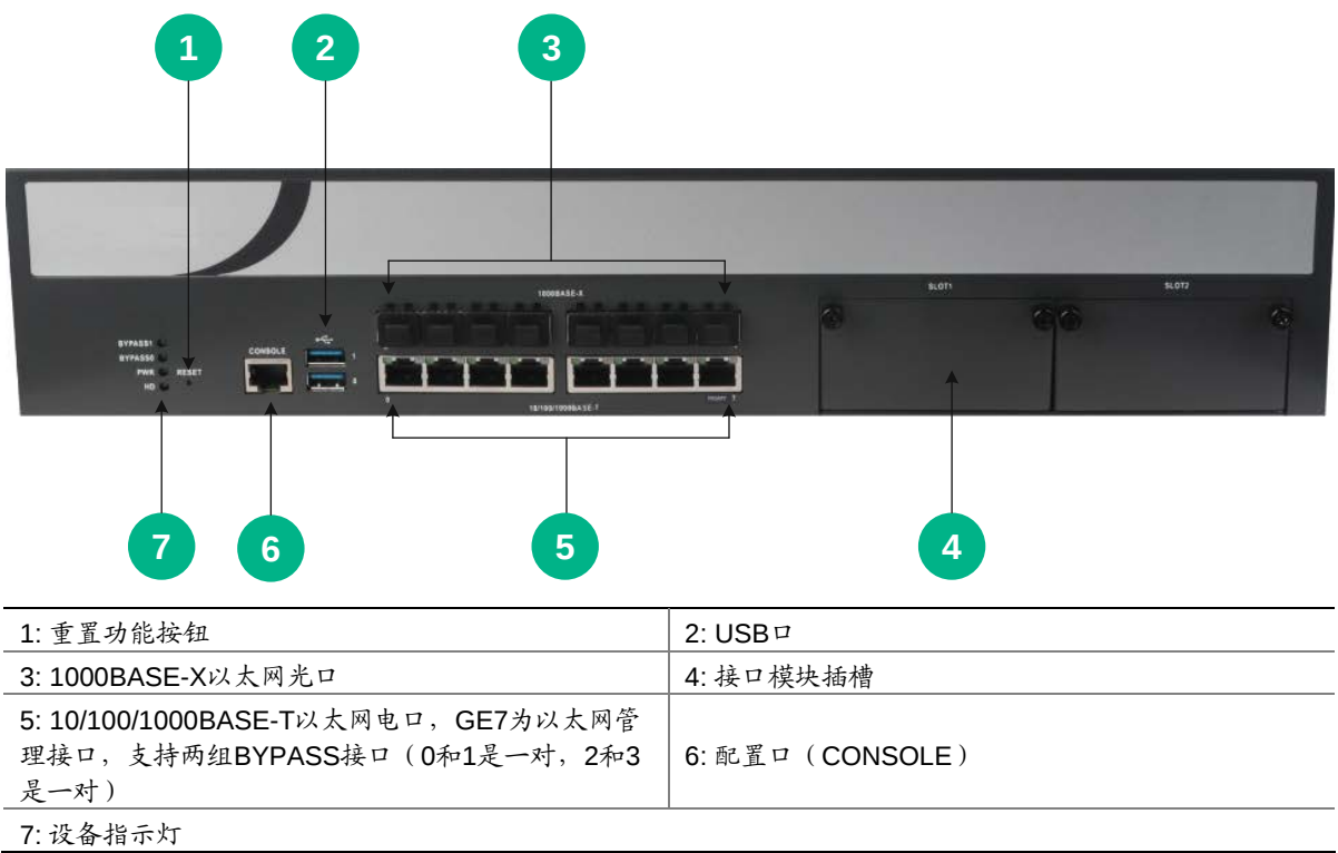
图A-1 UNIS W2000-G30 设备前视图
