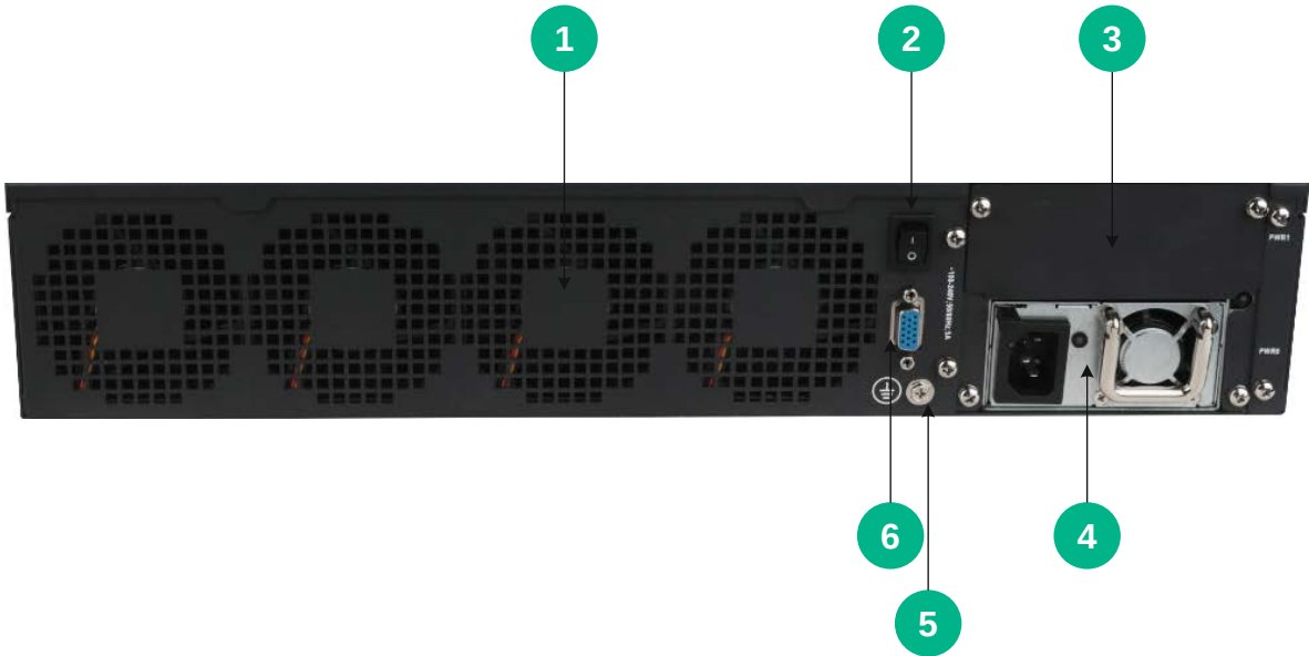
图A-4 UNIS W2000-G50 设备后视图
